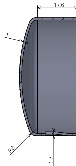
断面図 S-S
